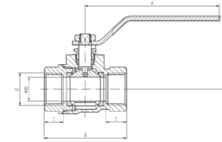
Plena (Ø D - completo/passagem de fluxo total)
