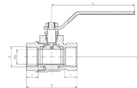
Pleno Heavy (Ø D - completo/passagem de fluxo total e alta pressão)
